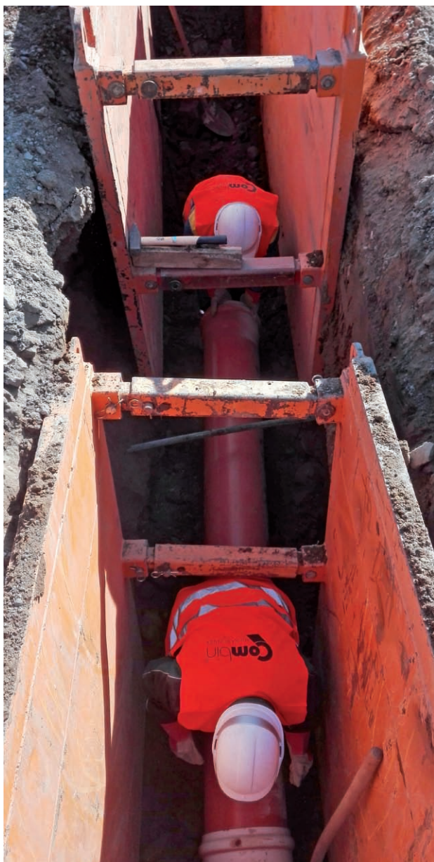
Medzibrodie nad Oravou - rozšírenie vodovodu a kanalizácie
